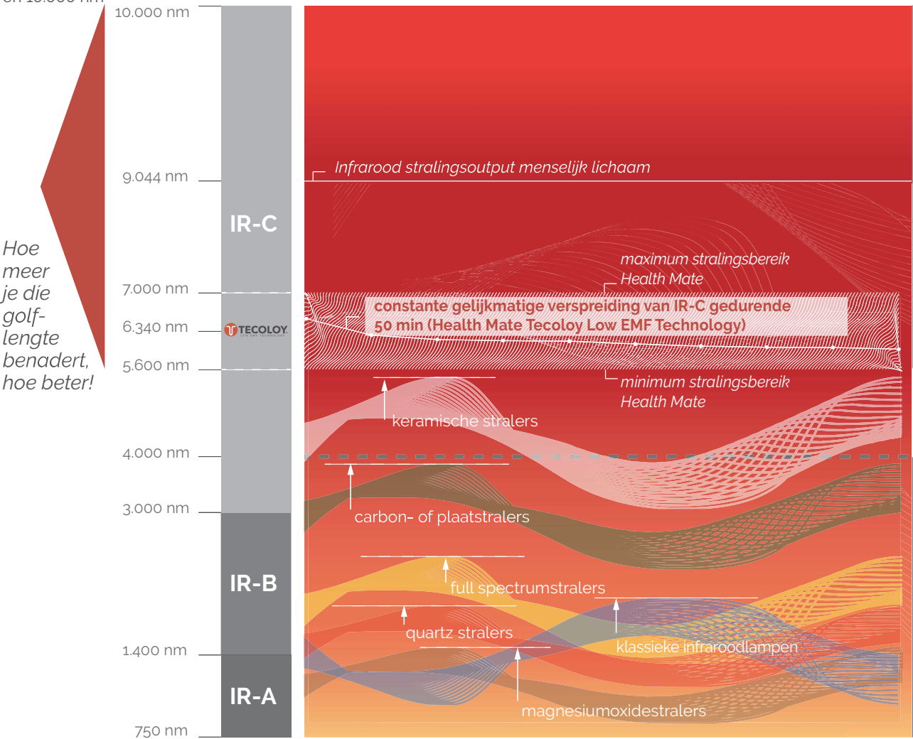
Spectrale emissies bij een constant maximaal stralingsvermogen
